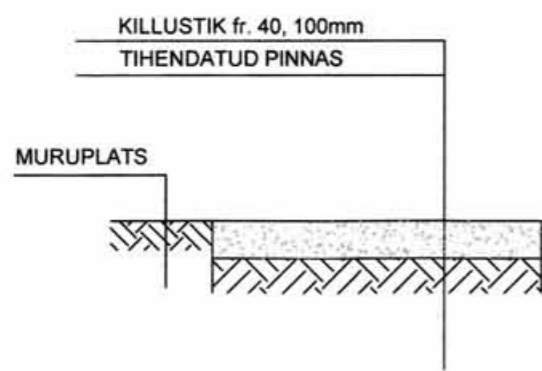
LÕIGE 1-1 M 1:40
