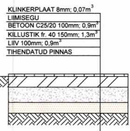
LÕIGE 3-3 M 1:40
