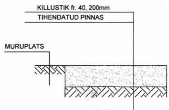
LÕIGE 2-2 M 1:40
