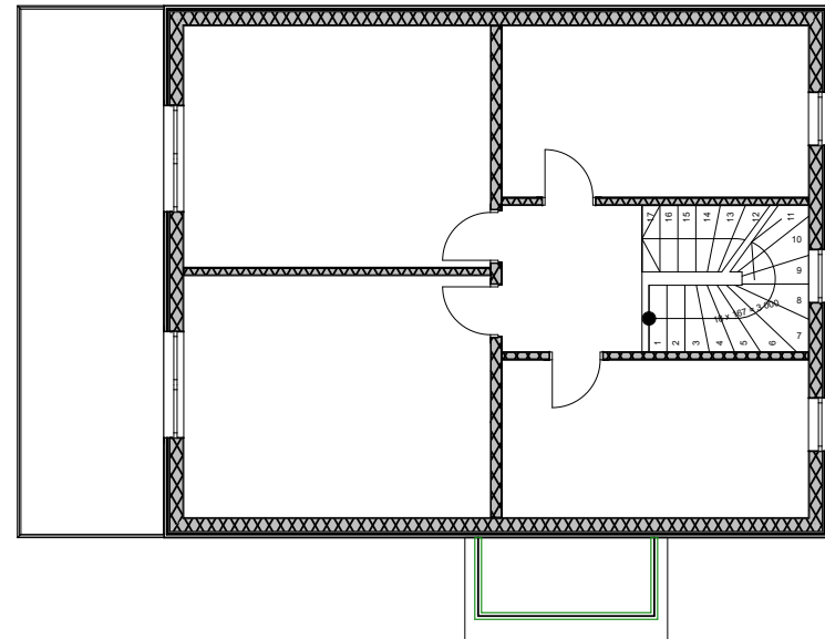
TEINE KORRUS
