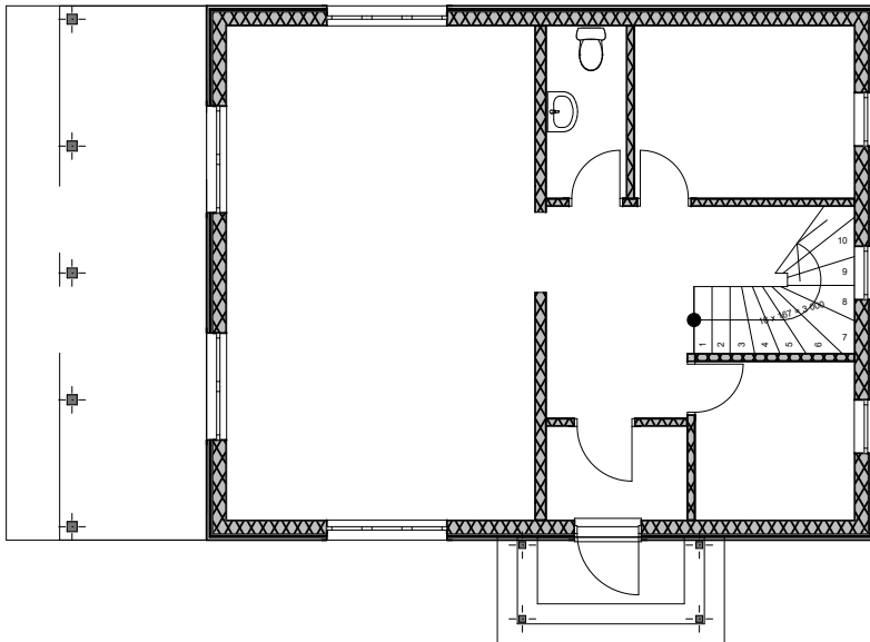
ESIMENE KORRUS
